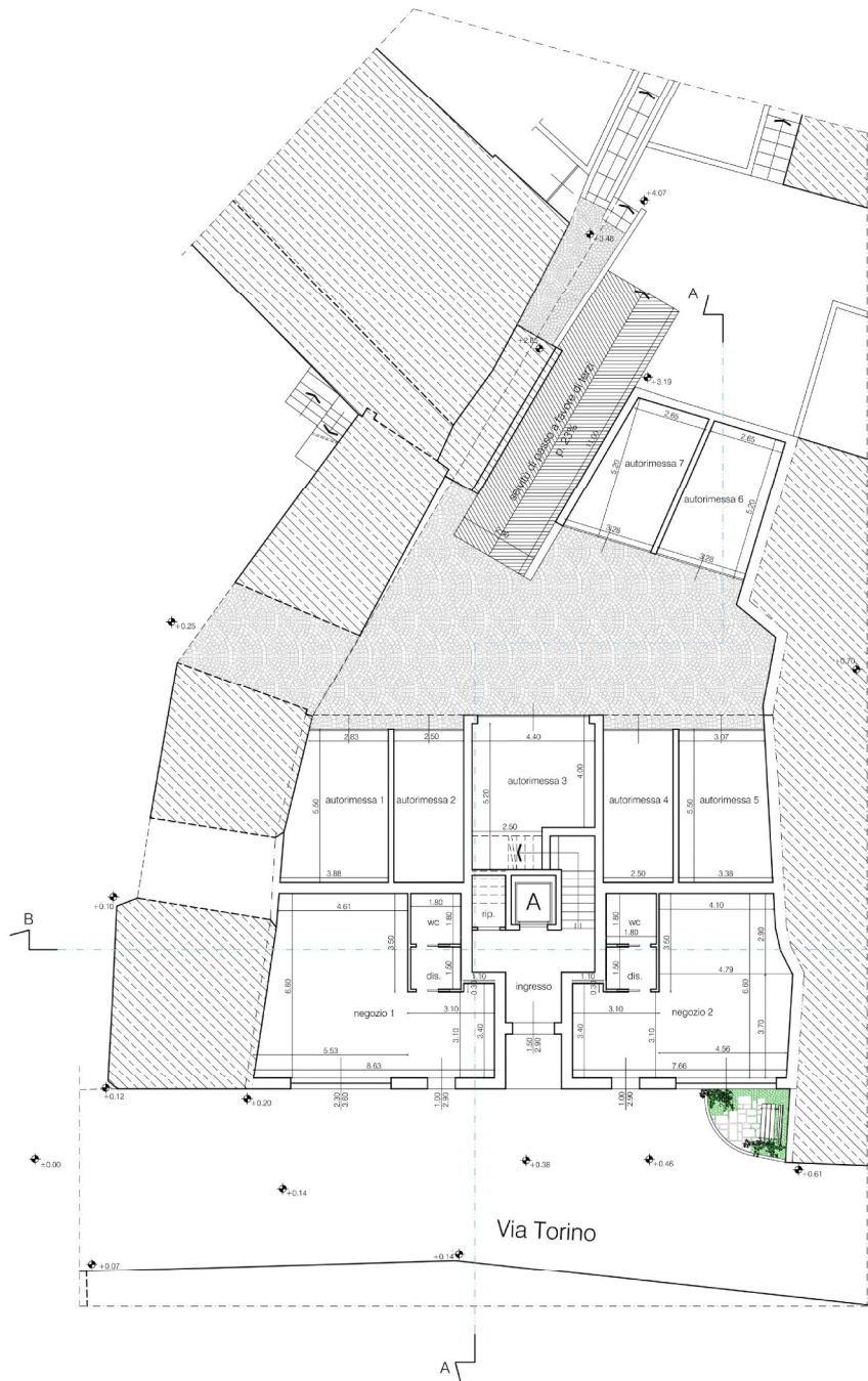
Piano Terreno sc. 1:100
